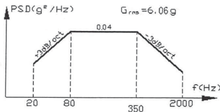
图1 随机振动验收试验条件
